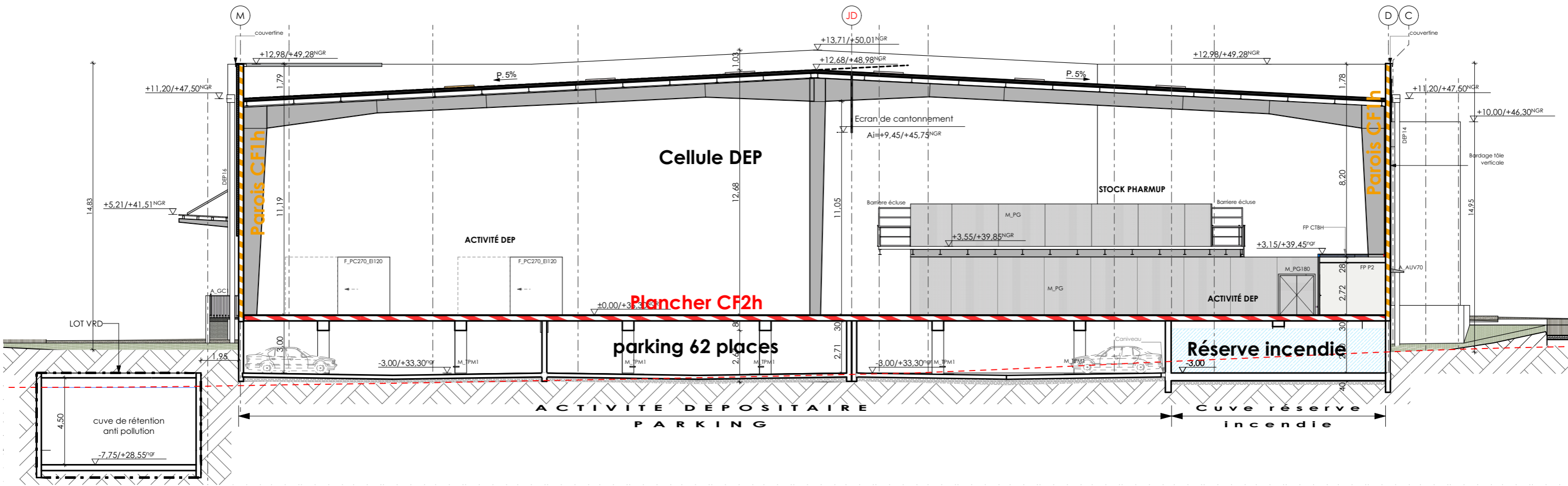
COUPE D
